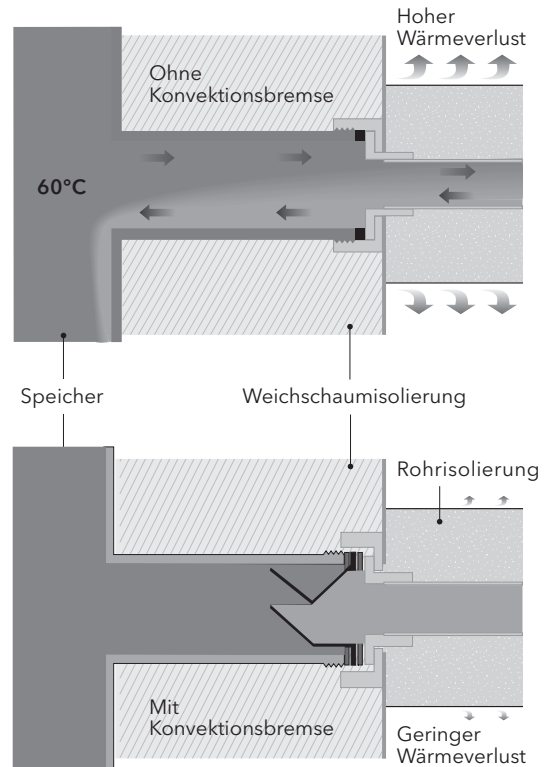
Bild 4 Wärmeverluste an Speicher-Rohranschlüssen ohne und mit CONVECTROL-Konvektionsbremse
